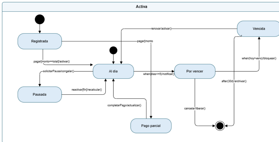
Figura 7: Máquina de Estados UML de la entidad Membresía (con estado compuesto).
