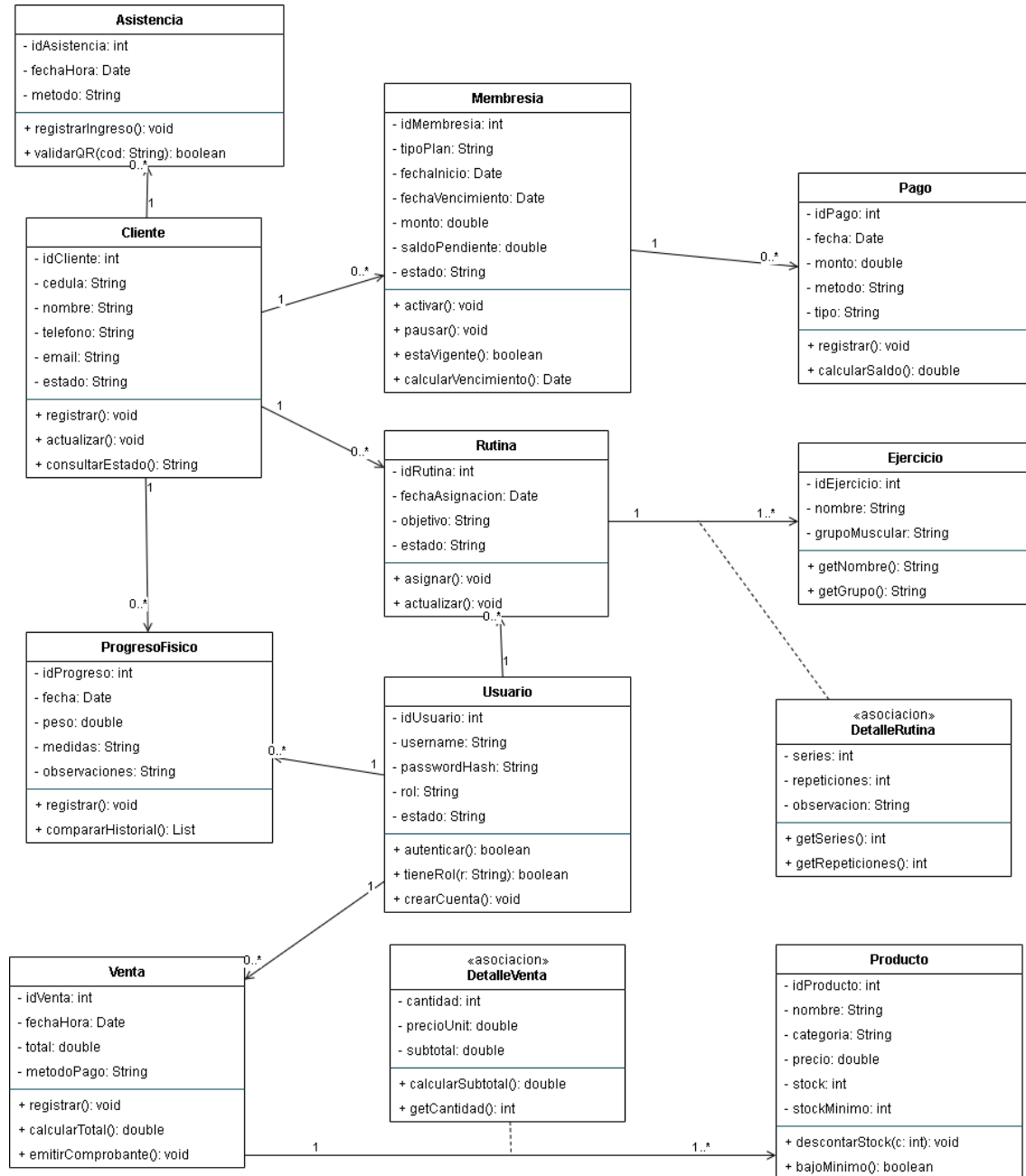
Figura 2: Diagrama de Clases UML derivado del modelo ER
